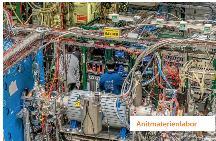
Versuchsanlage
